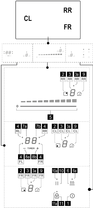
Bedienfeld Mod.603
