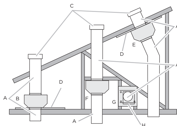
A. Conduit rond B. Fixation au dessus des solives de plafond C. Bouches de décharge par le toit D. Contreplaqué
