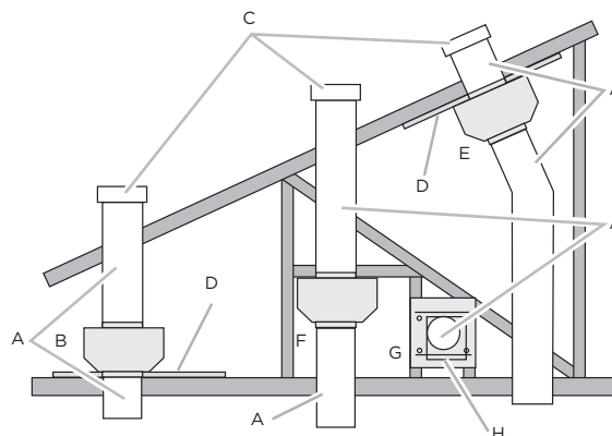
A. Ducto B. Montaje encima de las vigas del techo. C. Boquillas de techo D. Tablaroca (opcional para algunas instalaciones) E. Montaje por debajo de las vigas del techo F. Monte desde travesaños atados a estructura. G. Ducto horizontal; Monte de de travesaños atados a estructura. H. Boquilla de pared
