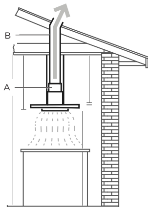
A. Transición redonda B. Ducto redondo
