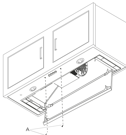
A. Tornillos - 4.2 x 15 mm (2)
