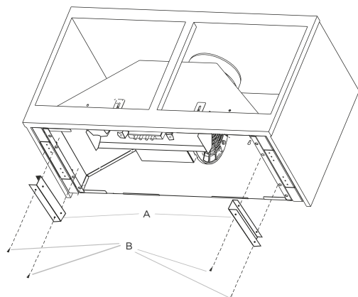
A. Soportes para panel inferior (2) B. Tornillos - 3.5 x 6.5 mm (4)
